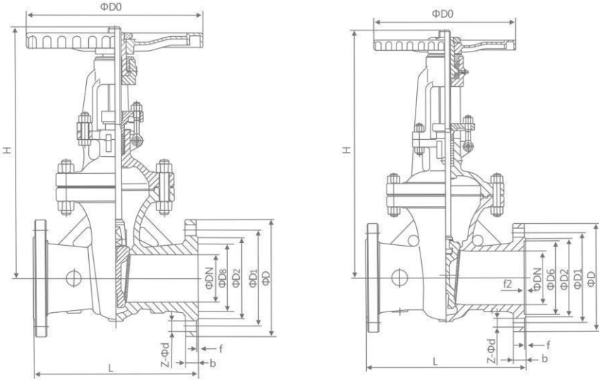
主要外形尺寸及连接尺寸Main external and connection dimensionJB/T79.2-1994JB/T79.4-1994
